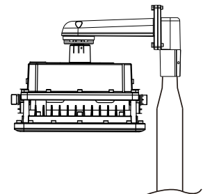
Montaje con Brazo en Poste
