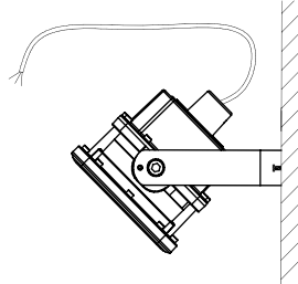
Montaje en pared, ángulo ajustable. Soporte Incluido.
