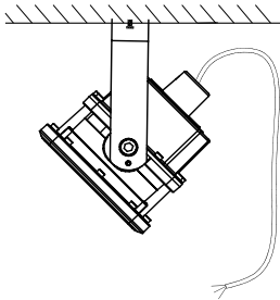
Montaje en techo, ángulo ajustable. Soporte Incluido.
